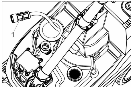
1 Filter färskvatten
